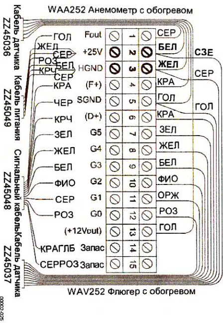
Рисунок 1 Стандартная схема WAC151 для WAA252 и WAV252
