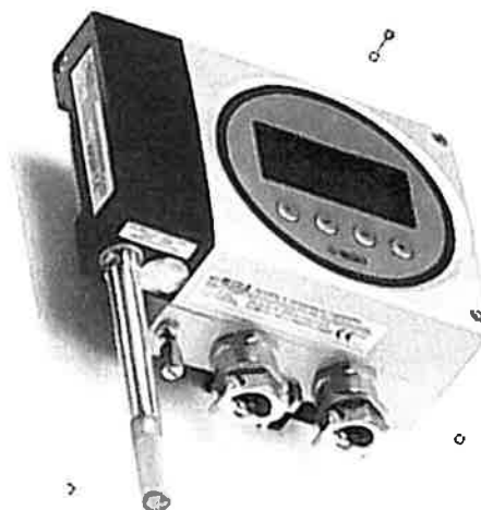
Рисунок 1. Внешний вид измерителя влажности и температуры НМТ360
