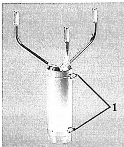
Рисунок 2. Схема пломбирования преобразователей WMT700. Пломбы на преобразователе – 1.
