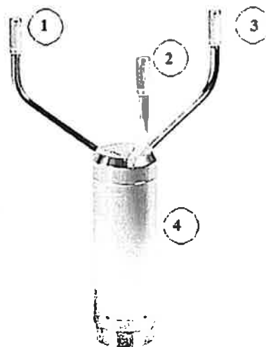
Рис. 1. Внешний вид преобразователей WMT700. Первичные преобразователи - 1, 2, 3 корпус – 4.
