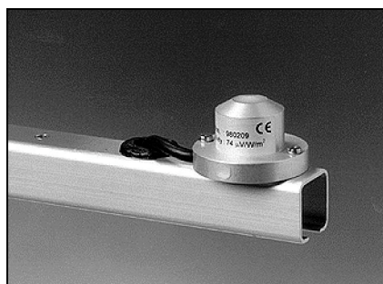
Рисунок 66 Пиранометр QMS101
