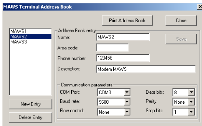
Рисунок 114 Записи адресной книги для подключения по модемной линии
