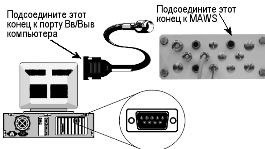
Рисунок 91 Подключение кабеля терминала
