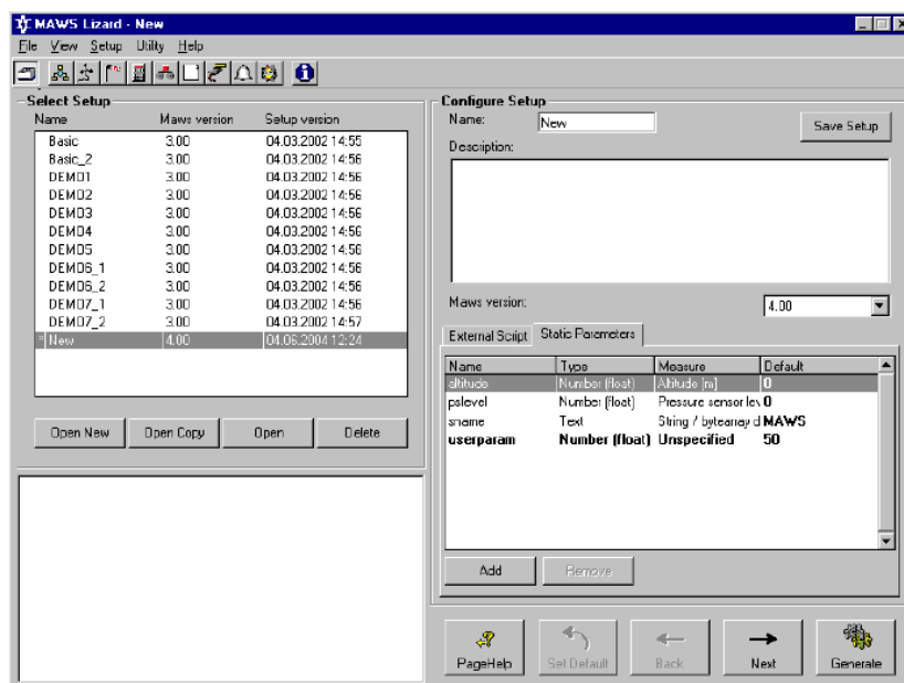
Рисунок 101 Setup Management (Управление настройками): Закладка Static Parameters (Статические параметры)
