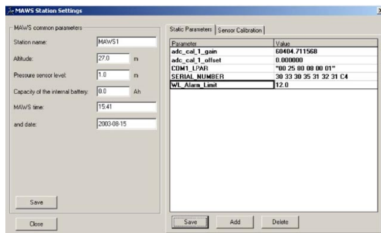
Рисунок 100 Окно установок станции MAWS
