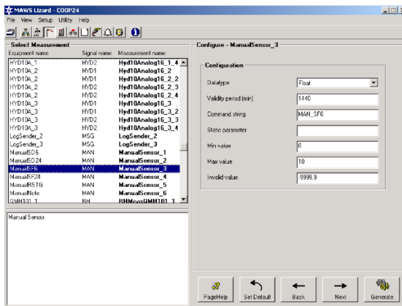
Рисунок 105 Конфигурация датчиков в программе MAWS Lizard
