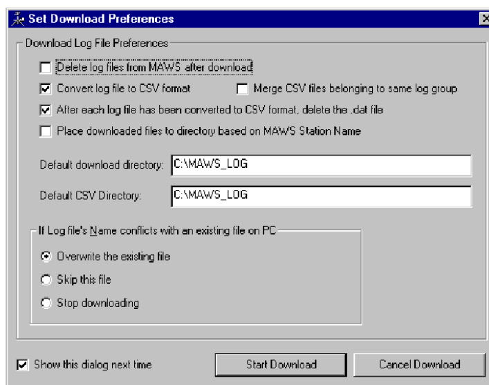
Рисунок 111 Окно Set Download Preferences
