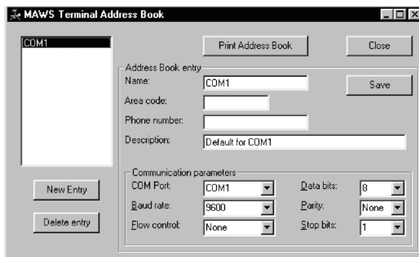
Рисунок 98 Окно Адресной книги
