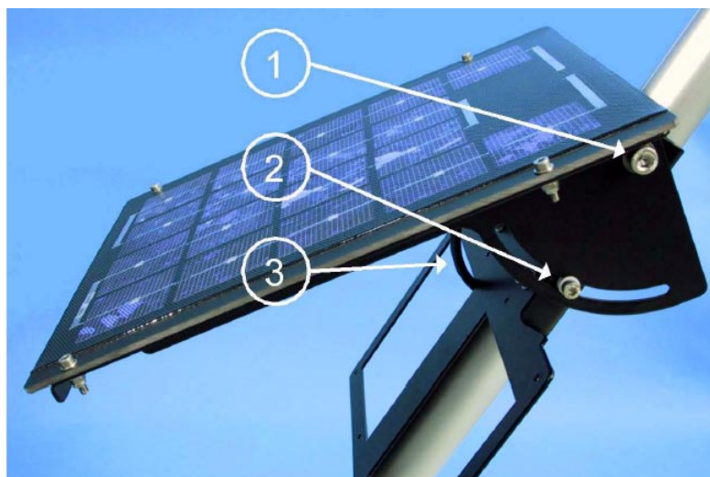
Рисунок 89 Настройка угла наклона солнечной панели
