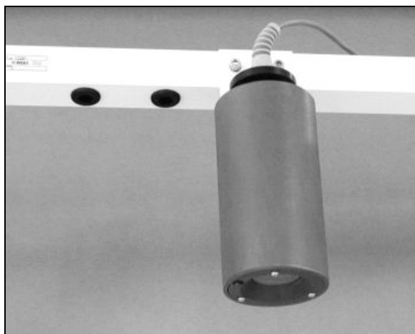
Рисунок 65 Датчик уровня снега DCU7210
