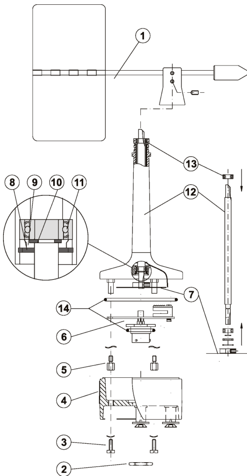
Рисунок 139 Блок WAV151
