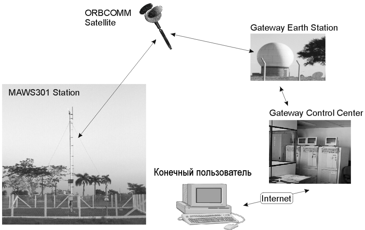
Рисунок 45 MAWS301 с ORBCOMM
