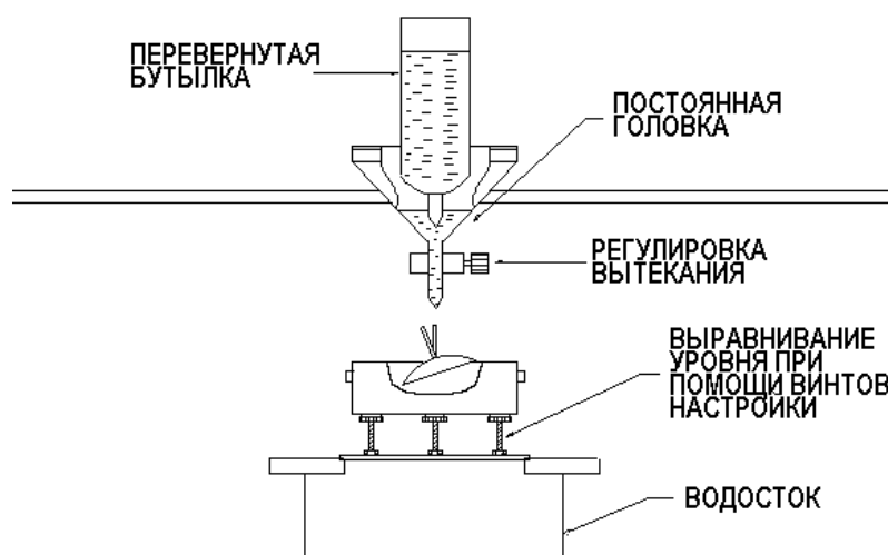
Рисунок 144 Динамическая калибровка (Постоянный напор)
