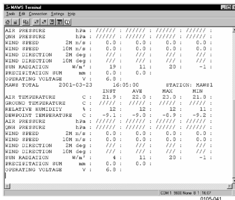
Рисунок 95 Отчет терминала MAWS
