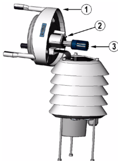
Рисунок 134 Замена модуля РТУ
