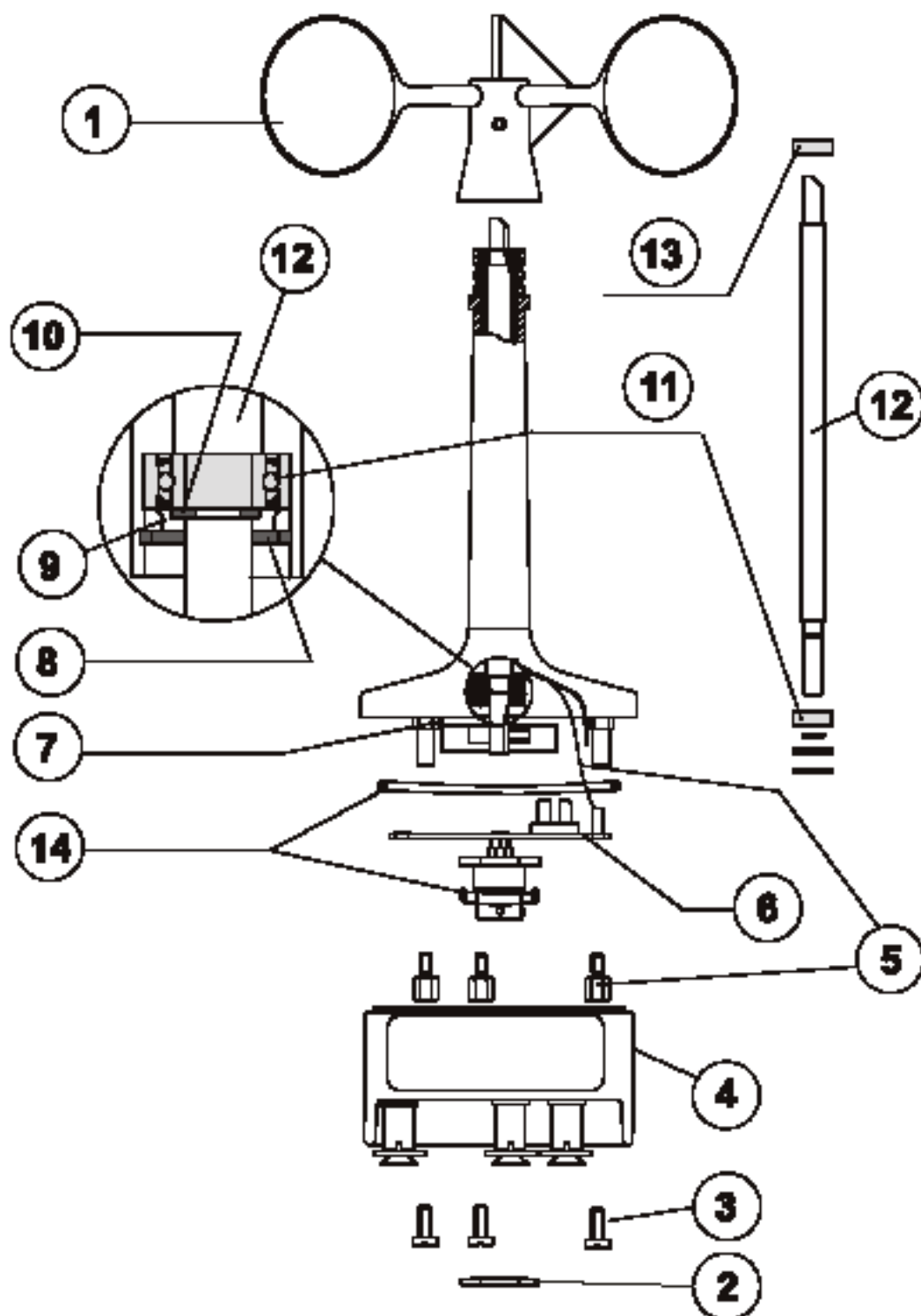
Рисунок 137 Блок WAA151
