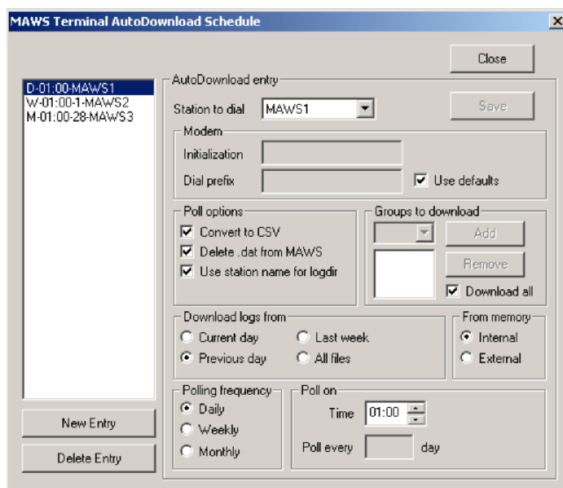
Рисунок 113 Окно AutoDownload Schedule (Расписание автозагрузки)
