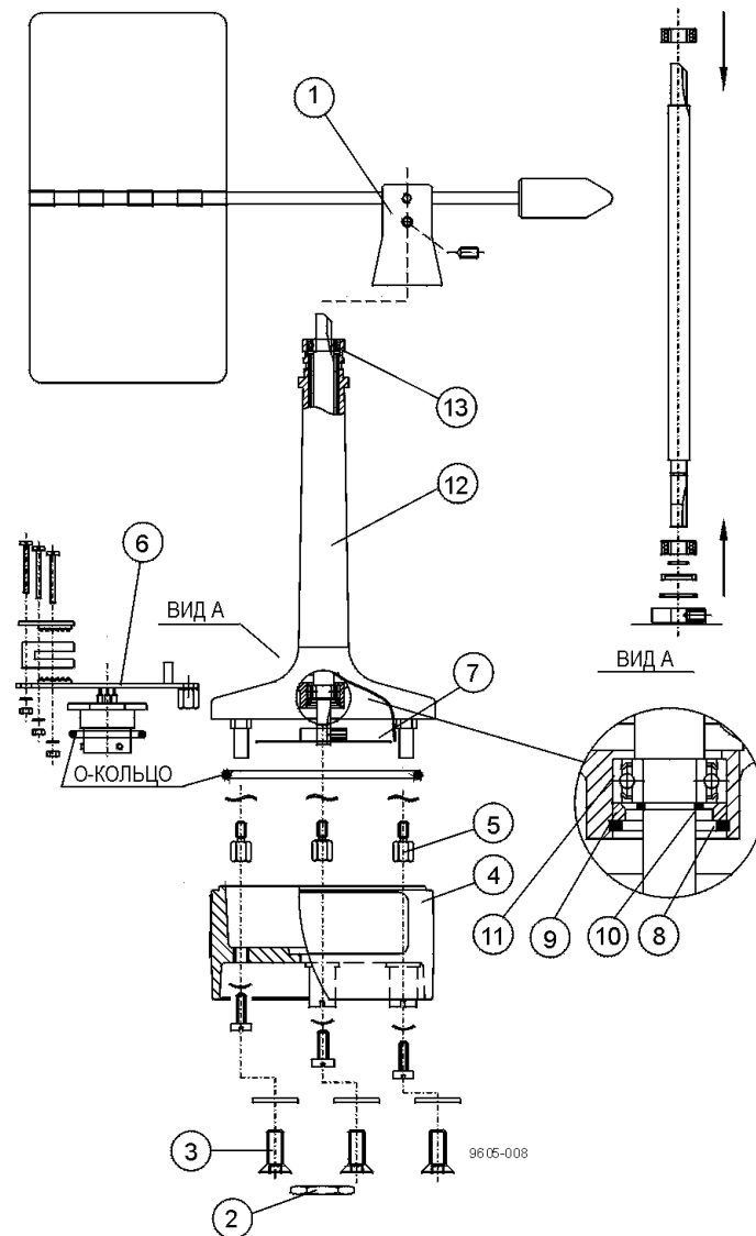
Рисунок 140 Блок WAV151
