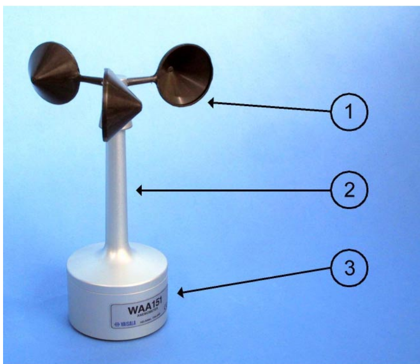
Рисунок 53 Анемоментр WAA151
