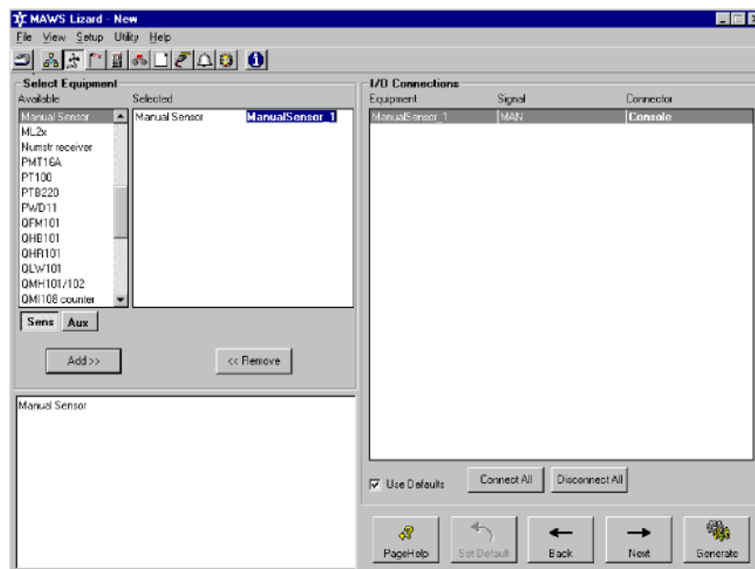
Рисунок 104 Создание ручных датчиков в программе MAWS Lizard
