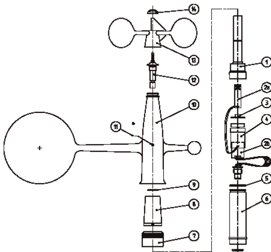
Рисунок 136 Состав датчика WMS
