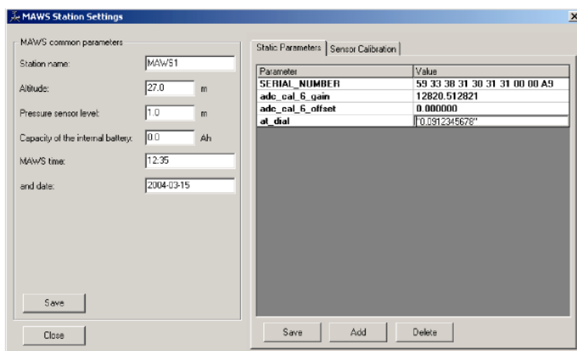
Рисунок 102 Окно Station Settings (Настройки станции) программы Maws Terminal
