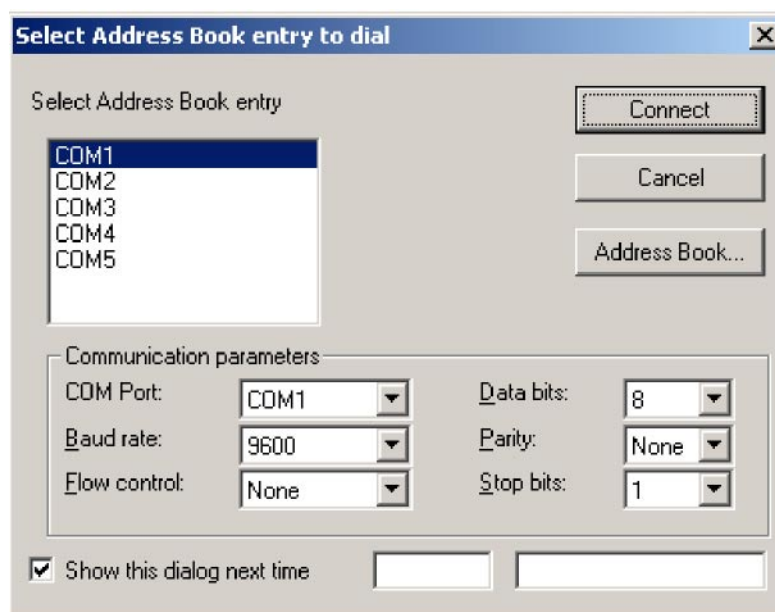
Рисунок 99 Окно Select Address Book Entry to Dial (Выберите запись Адресной книги для набора)
