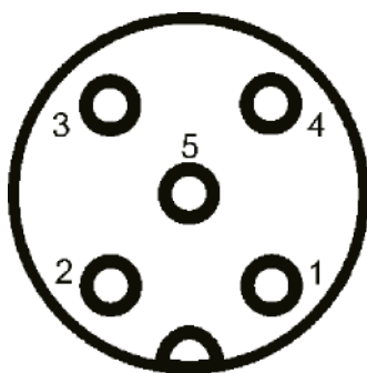
Рисунок 92 COM0 контакты разъема терминала
