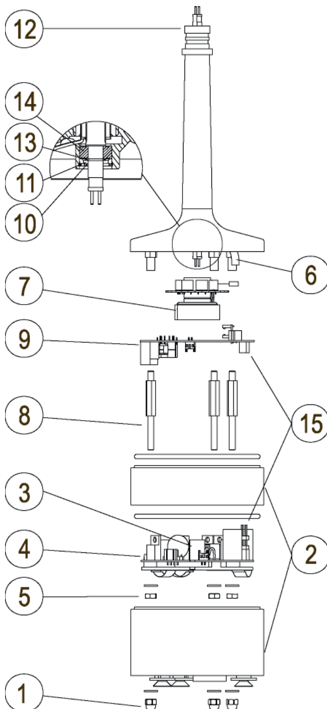
Рисунок 138 Блок WAA252
