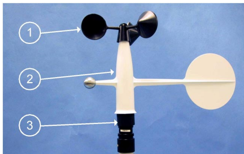
Рисунок 52 Комбинированный датчик ветра
