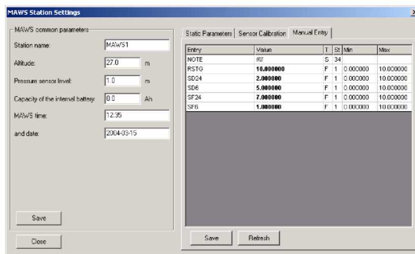
Рисунок 106 Закладка Manual Entry (Ручной ввод)
