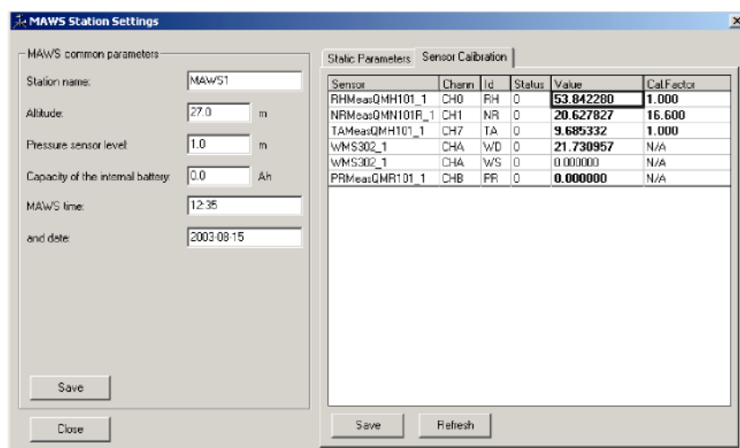
Рисунок 103 Окно MAWS Station Settings (Настройки станции MAWS: закладка Sensor Calibration (Калибровка датчика))
