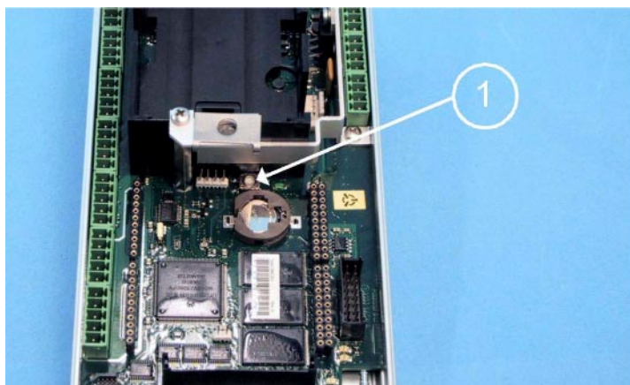
Рисунок 125 Кнопка перезапуска логгера
