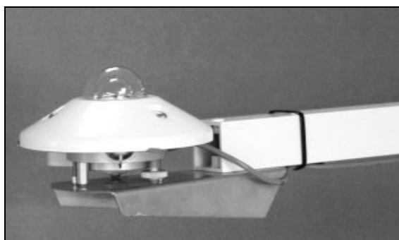
Рисунок 68 Пиранометр SM6B
