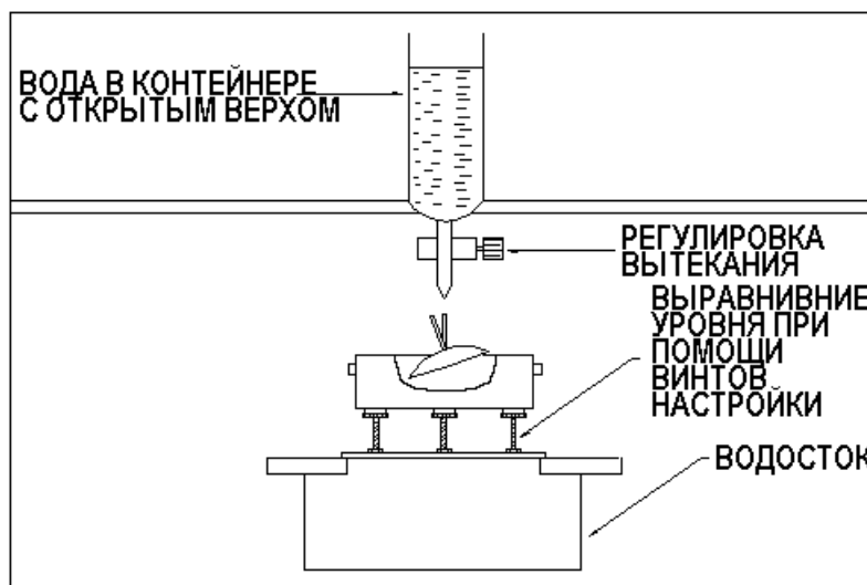
Рисунок 143 Динамическая калибровка
