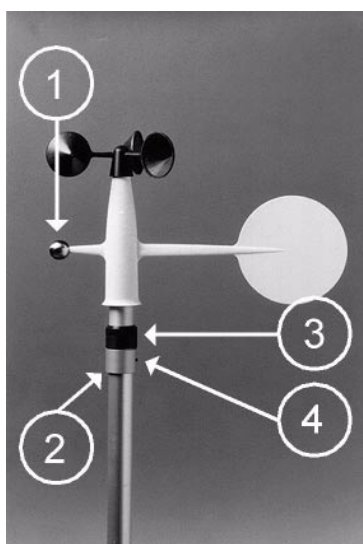
Рисунок 88 Выравнивание флюгарки
